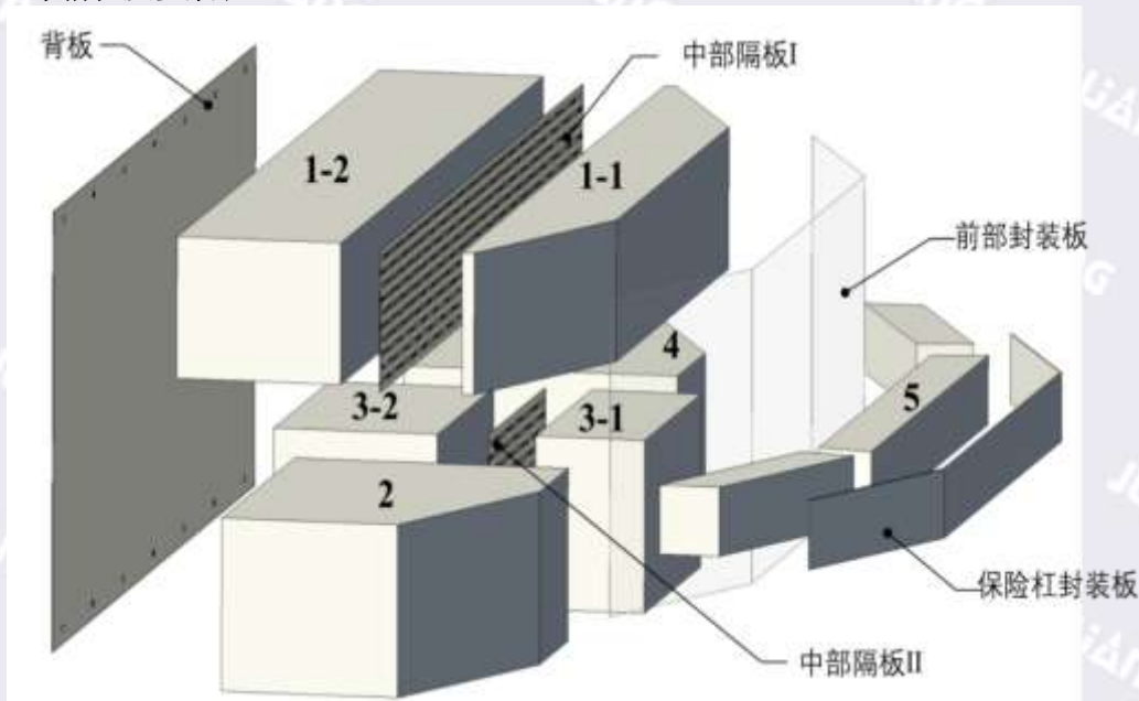
图 1 产品装备爆炸图
